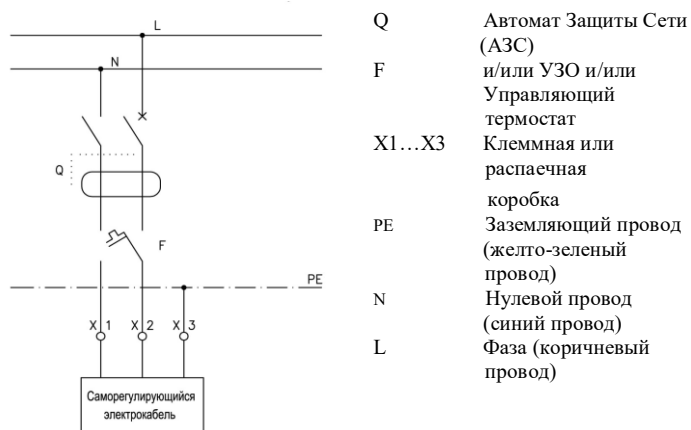
Рис. 5. Схема подключения электрообогрева кровельной воронки HL62.1H к электрической сети.
