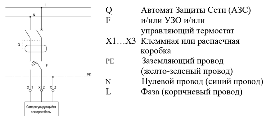
Рис. 5. Схема подключения электрообогрева кровельной воронки HL64.1 к электрической сети.
