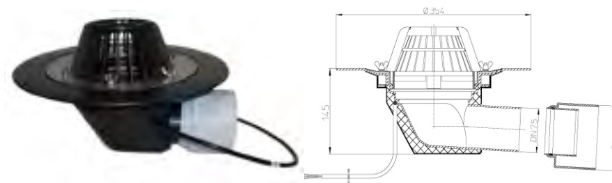
Рис. 1. Кровельная воронка HL64.1
