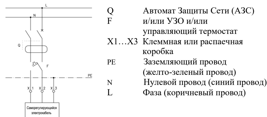
Рис. 5. Схема подключения электрообогрева кровельной воронки HL64.1 к электрической сети.
