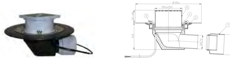
Рис. 1. Кровельная воронка HL64.1B
