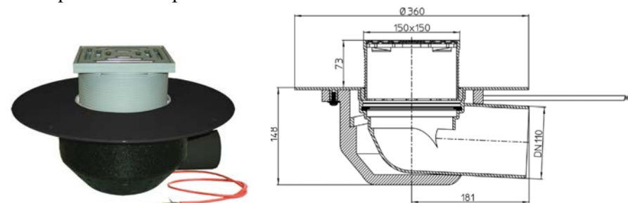
Рис. 1. Кровельная воронка HL64.1BF.
