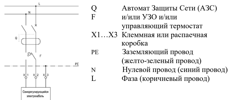
Рис. 3. Схема подключения электрообогрева кровельной воронки HL64.1BF к электрической сети.
