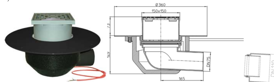
Рис. 1. Кровельная воронка HL64.1BF.
