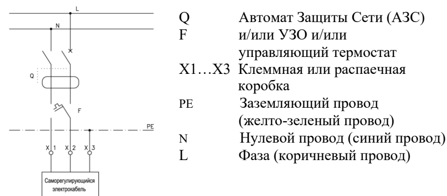
Рис. 5. Схема подключения электрообогрева кровельной воронки HL64.1BH к электрической сети.
