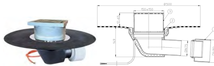
Рис. 1. Кровельная воронка HL64.1BH
