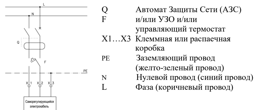
Рис. 5. Схема подключения электрообогрева кровельной воронки HL64.1H к электрической сети.
