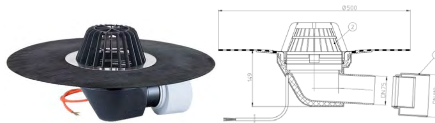
Рис. 1. Кровельная воронка HL64.1H
