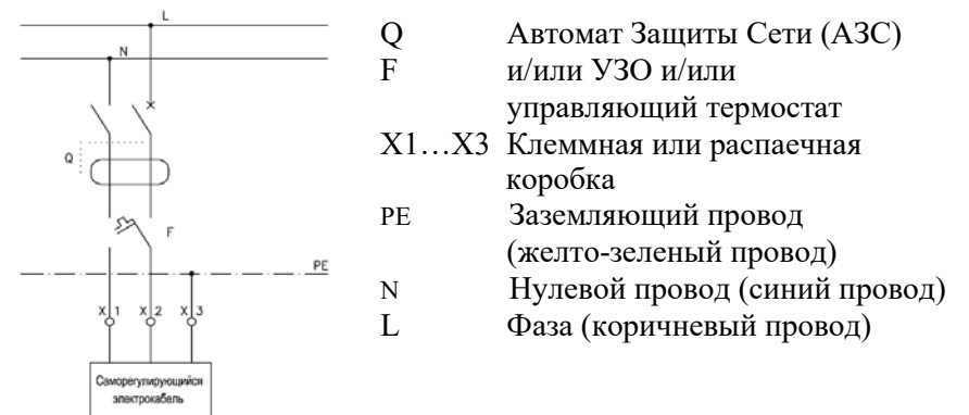
Рис. 3. Схема подключения электрообогрева кровельной воронки HL64.1P к электрической сети.
