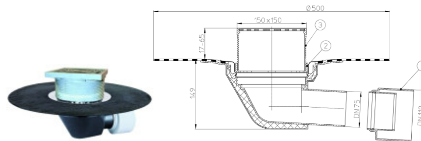
Рис. 1. Кровельная воронка HL64BH
