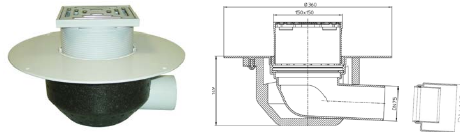
Рис. 1. Кровельная воронка HL64BP.
