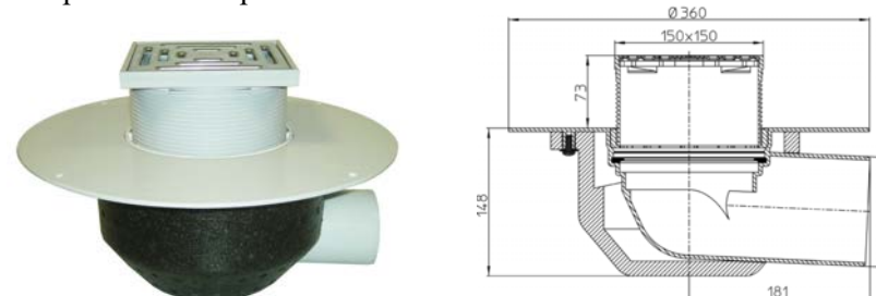
Рис. 1. Кровельная воронка HL64BP.
