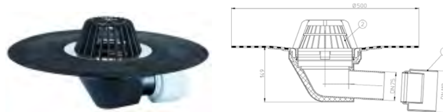
Рис. 1. Кровельная воронка HL64H
