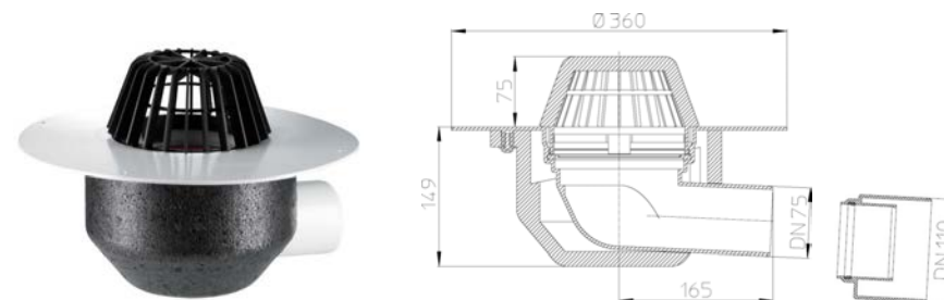
Рис. 1. Кровельная воронка HL64P.
