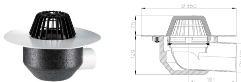
Рис. 2. Кровельная воронка HL64P/1.
